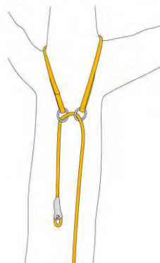
Fig. 8 - Ancoraggio passante per corda raddoppiata
